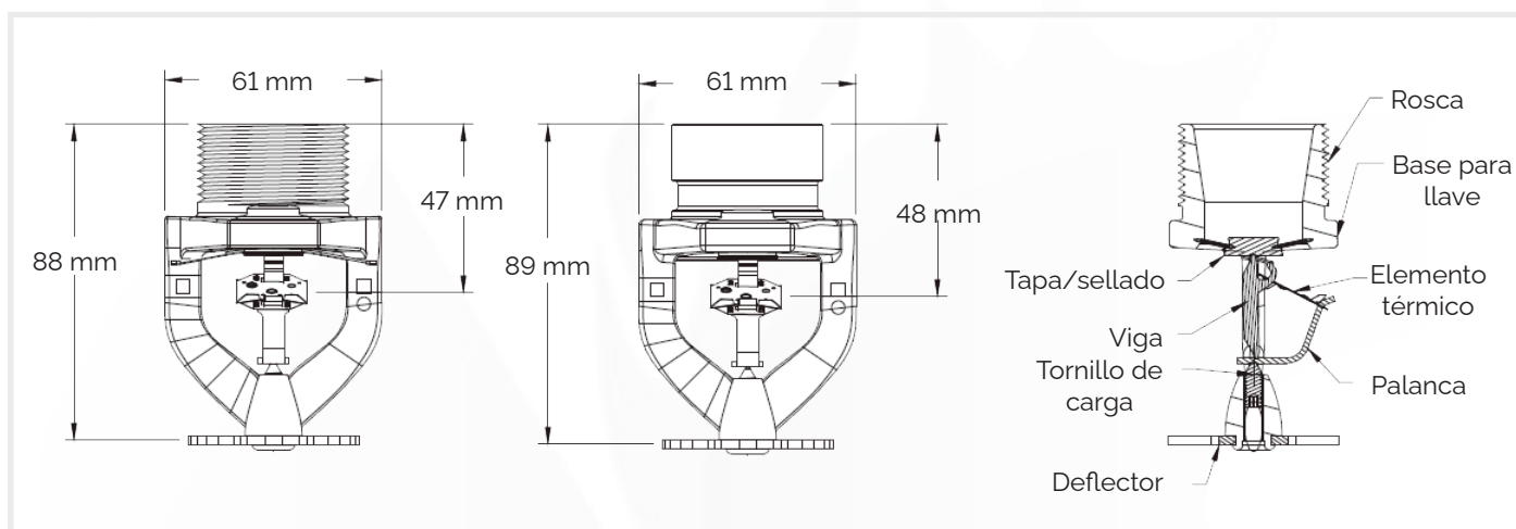
FIGURA 1: Dimensiones y componentes del Sprinkler M336
