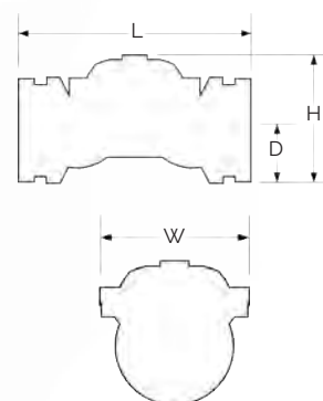
Figura 3: Plano conexión embreada.
