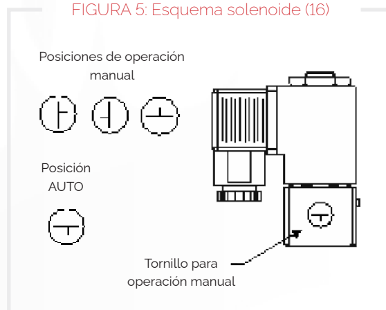
FIGURA 5: Esquema solenoide (16)
