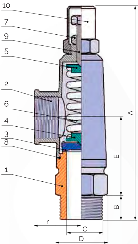
FIGURA 1: Componentes y dimensiones
