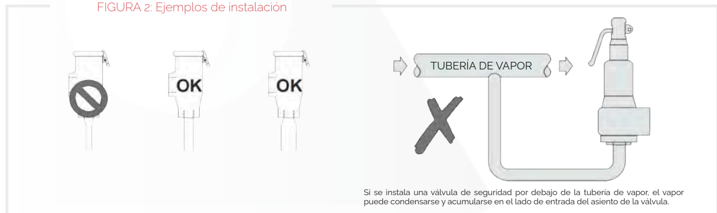
FIGURA 2: Ejemplos de instalación
