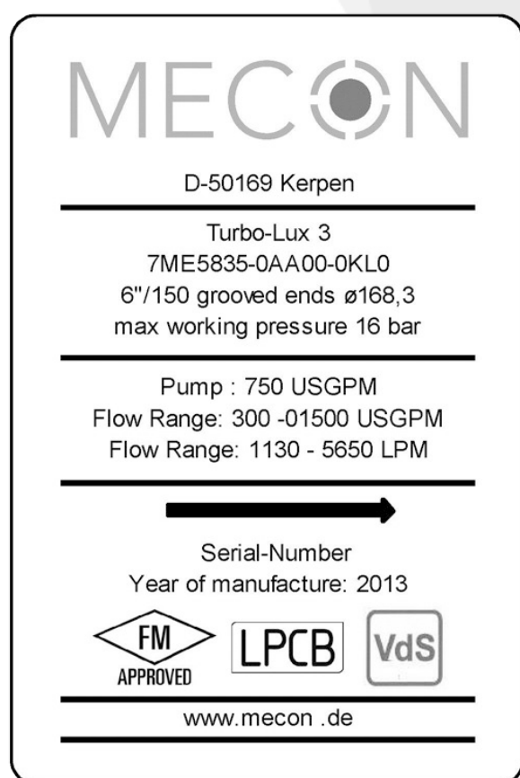
Fig. 3: Placa de características del diafragma de medición.
