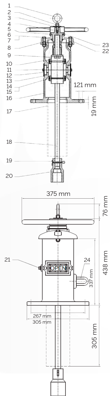
FIGURA 2: Dimensiones
