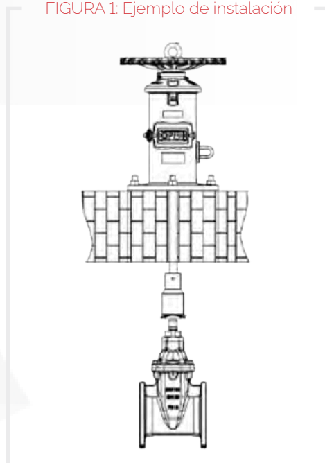
FIGURA 1: Ejemplo de instalación
