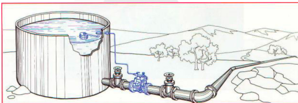
Esquema 14: Instalación de válvula de control de nivel.
