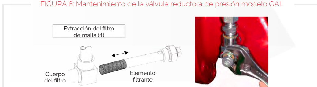
FIGURA 8: Mantenimiento de la válvula reductora de presión modelo GAL
