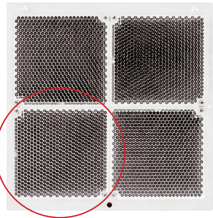
Reflector 50-100 m
