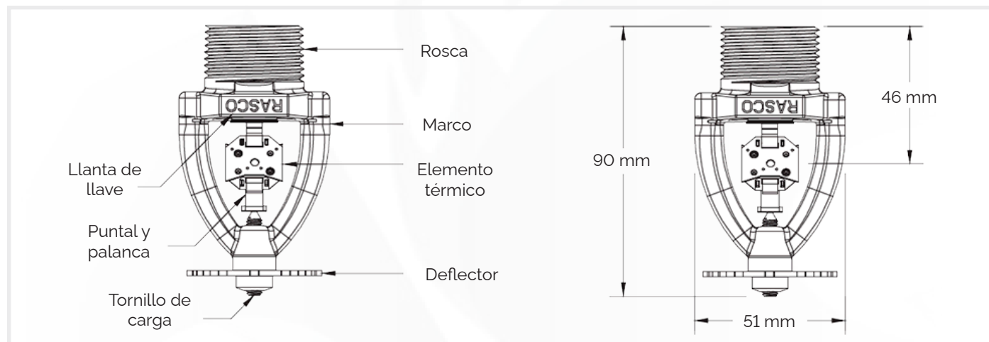
FIGURA 2: Sprinkler N252EC con embellecedor empotrado modelo FP
