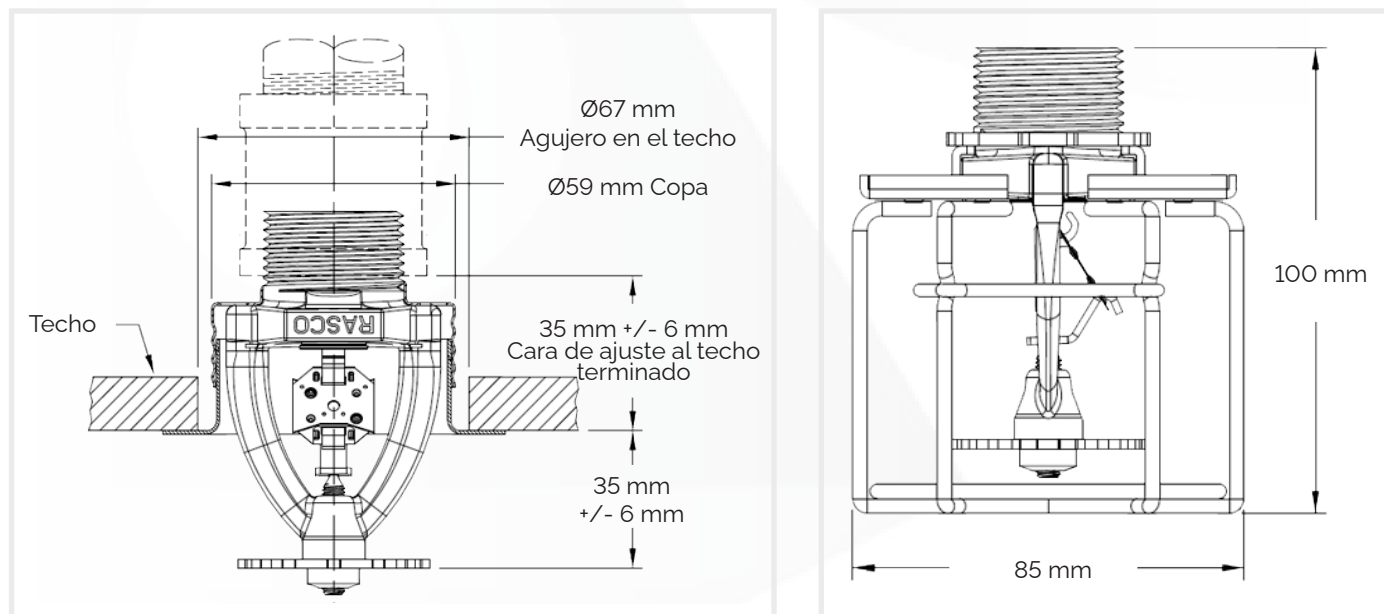
FIGURA 2: Sprinkler N252EC con embellecedor empotrado modelo FP
