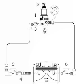
FIGURA 2: Componentes del sistema de control
