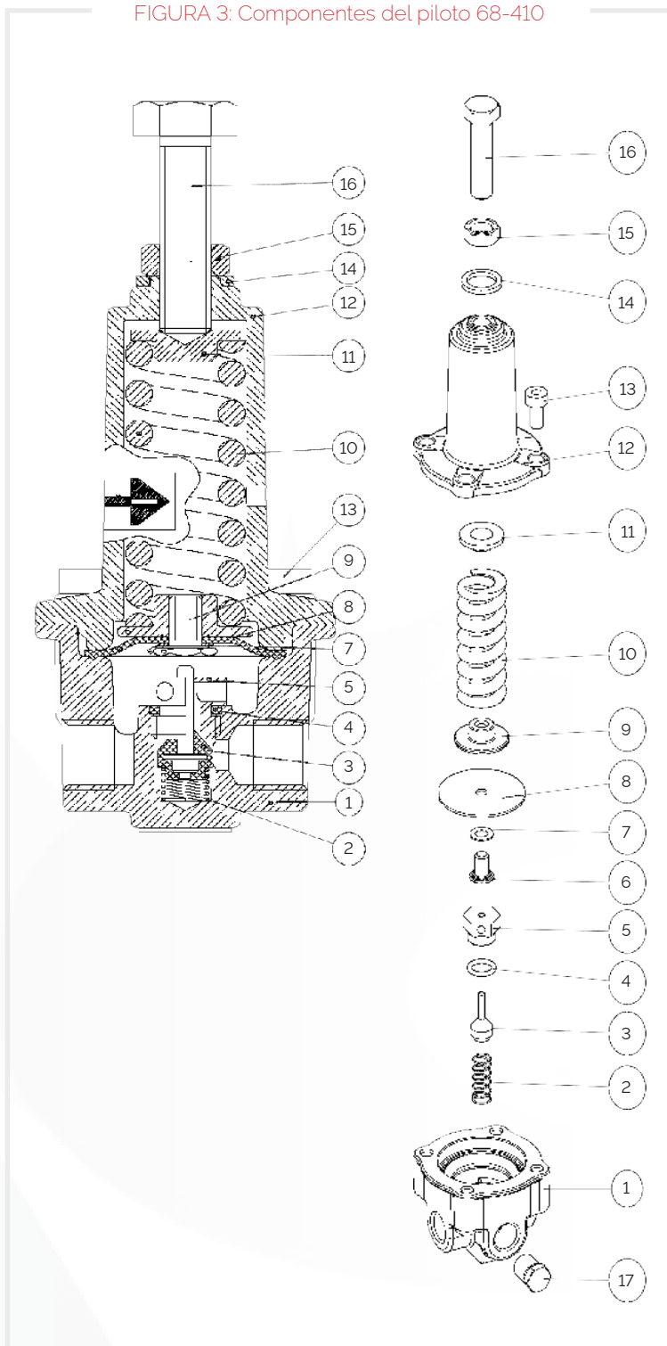
FIGURA 3: Componentes del piloto 68-410
