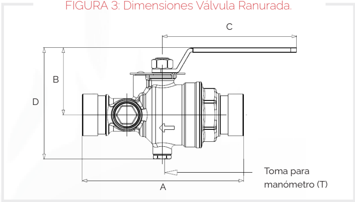
FIGURA 3: Dimensiones Válvula Ranurada.
