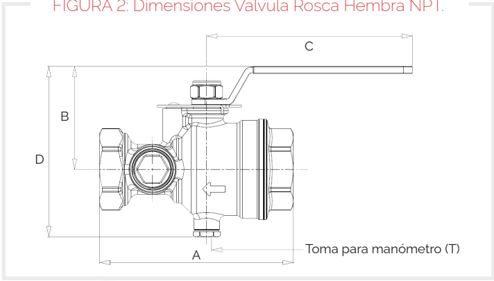
FIGURA 2: Dimensiones Válvula Rosca Hembra NPT.
