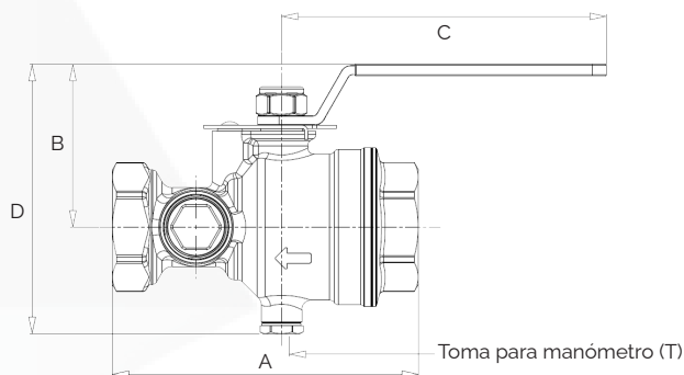
FIGURA 1: Dimensiones Válvula Rosca Hembra BSP.
