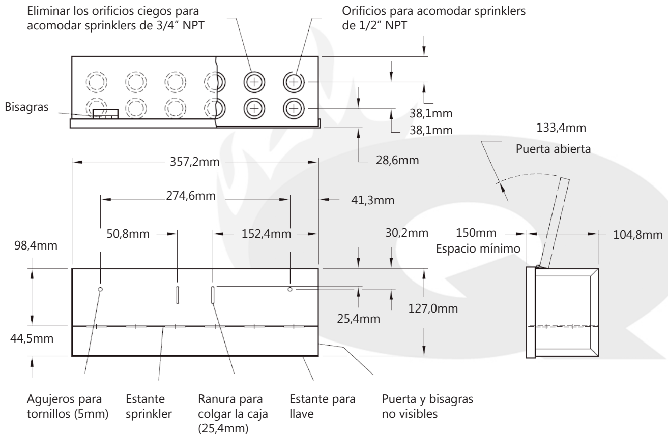
Figura 3. Caja de 6 sprinklers ESFR.
