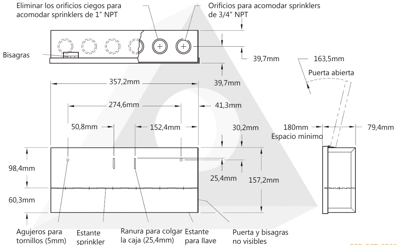
Figura 3. Caja de 6 sprinklers ESFR.
