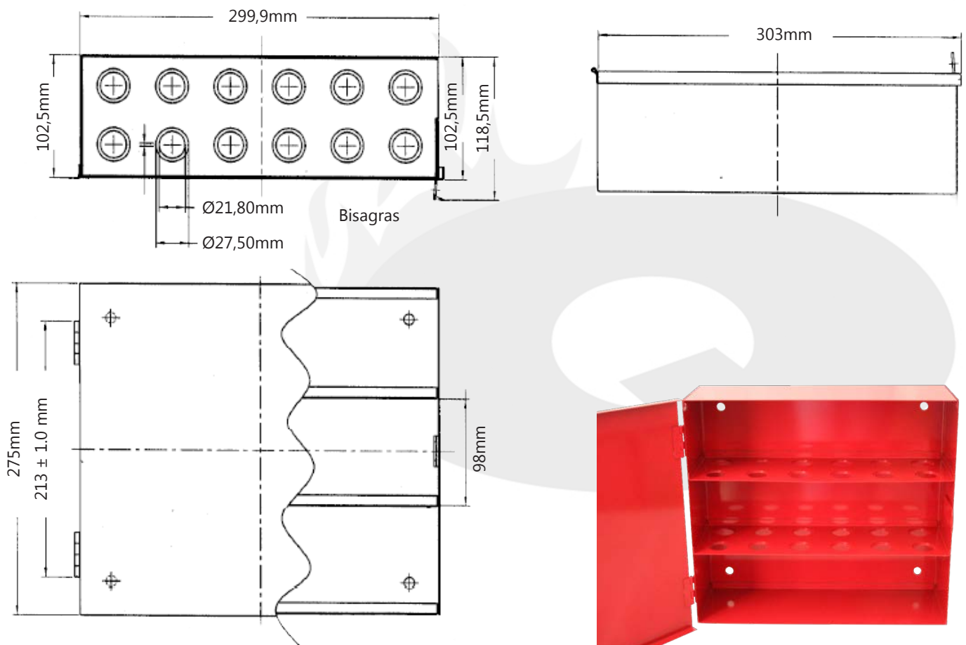
Figura 4. Caja de 24 sprinklers.
