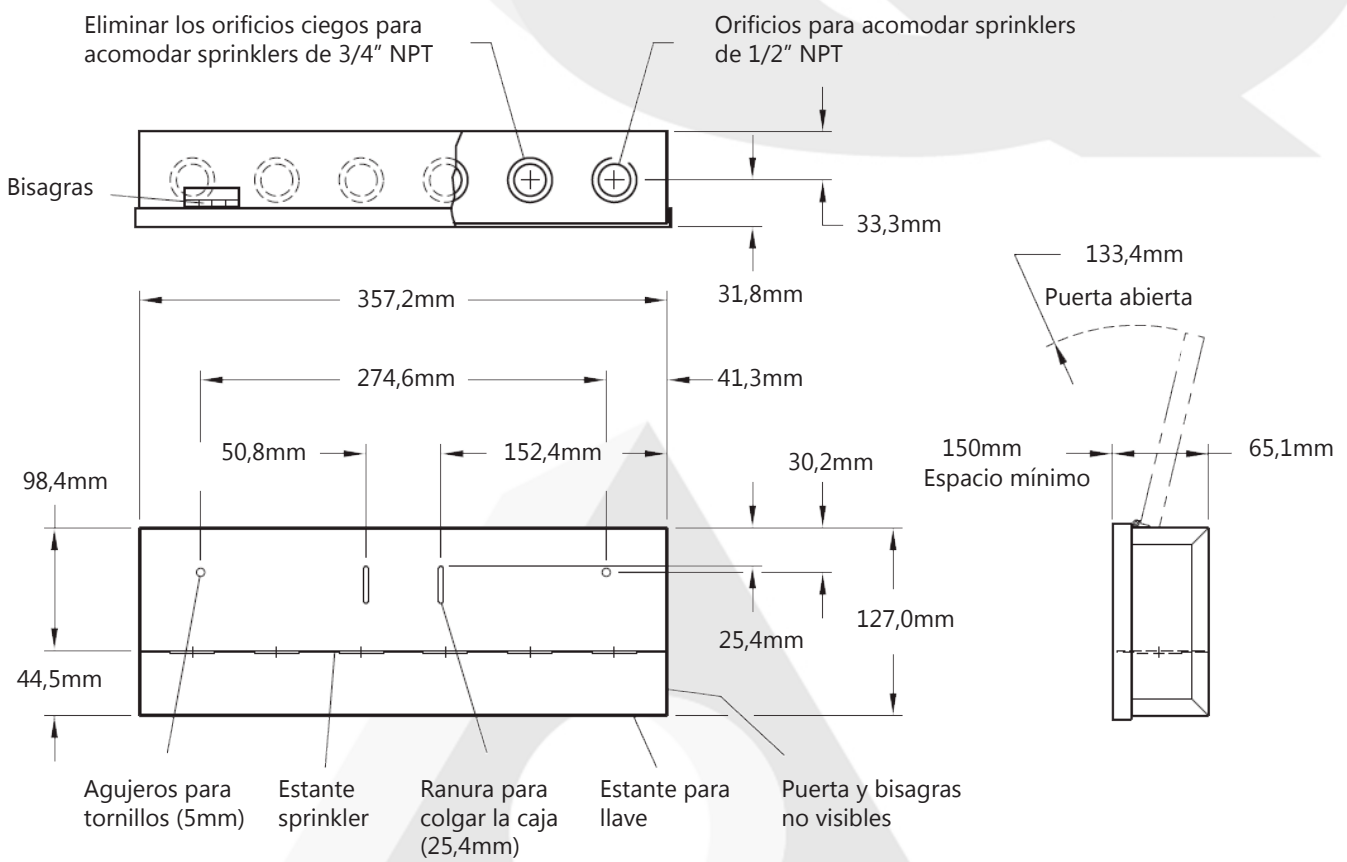
Figura 1. Caja de 6 sprinklers.
