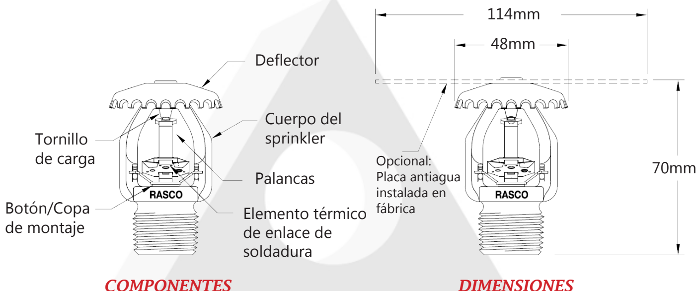
Figura 1 - Dimensiones y componentes del modelo GL112 montante
