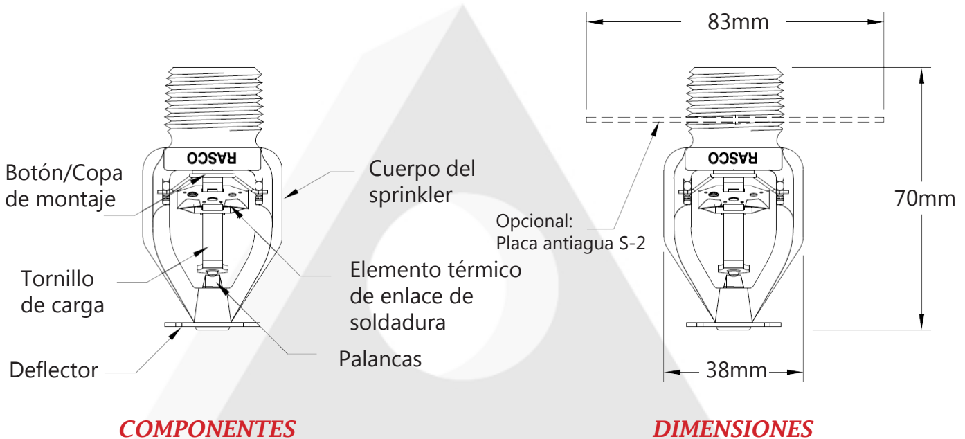
Figura 2 - Dimensiones y componentes del modelo GL112 colgante
