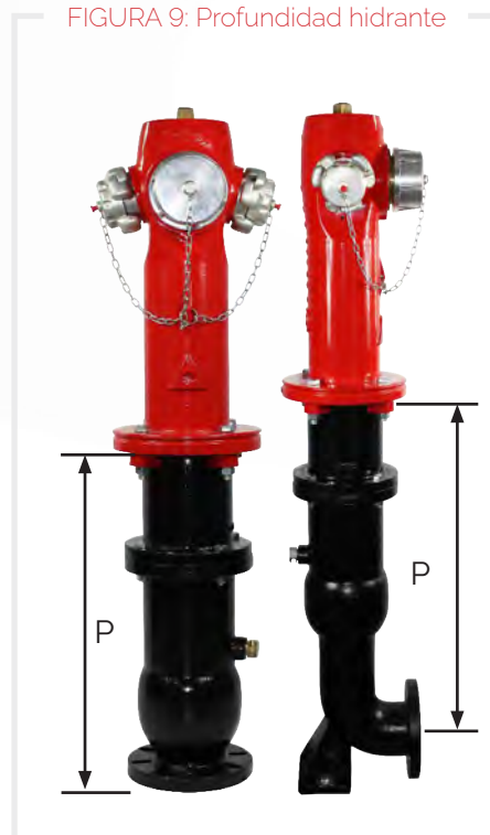
FIGURA 9: Profundidad hidrante
