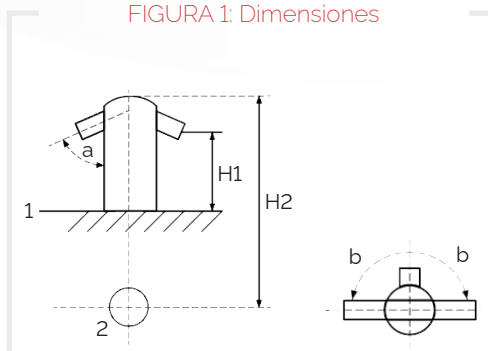
FIGURA 1: Dimensiones
